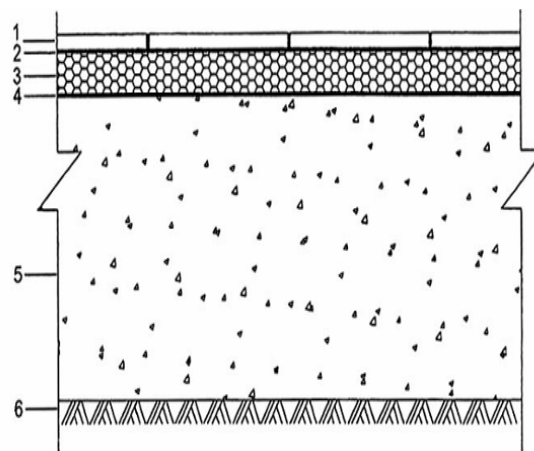
Hình 1 - Cấu tạo các lớp nền nhà chống nồm
